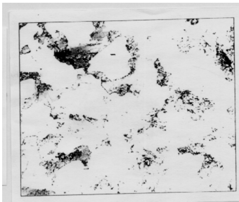
شکل 7 ساختار فولاد هایپوئوتکتوید متشکل از فریت پرویوتکتوید و پرلیت
