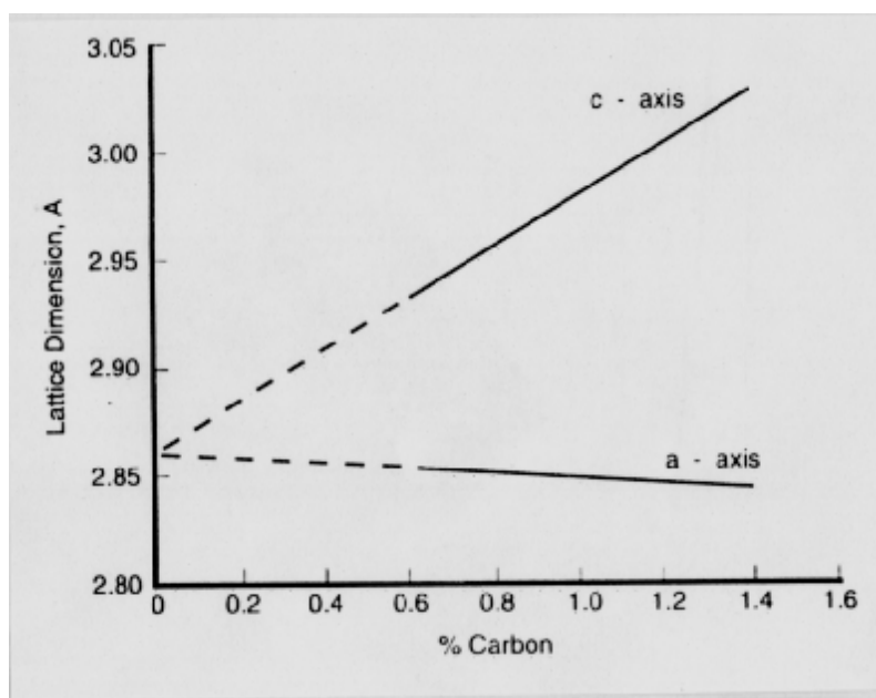
شکل 10 تاثیر اعوجاج روی ساختار bct به دلیل میزان کربن محور a و محور c در شکل 9-4 معرفی شده اند.
