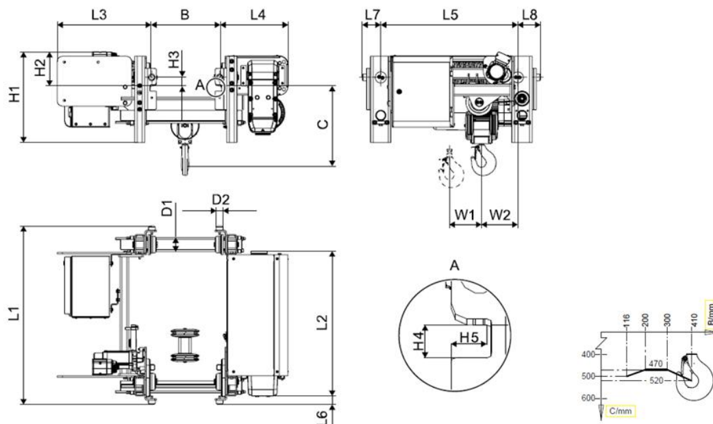
3.2t*6m Hoist Dimensions - 3.2 吨*6 米葫芦尺寸
